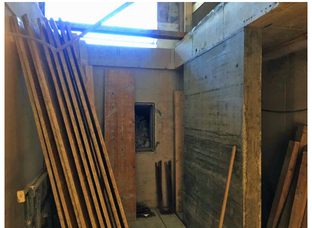
Ebnet 2, Untergeschoss: Neue Betonwand Aufzugsschacht
